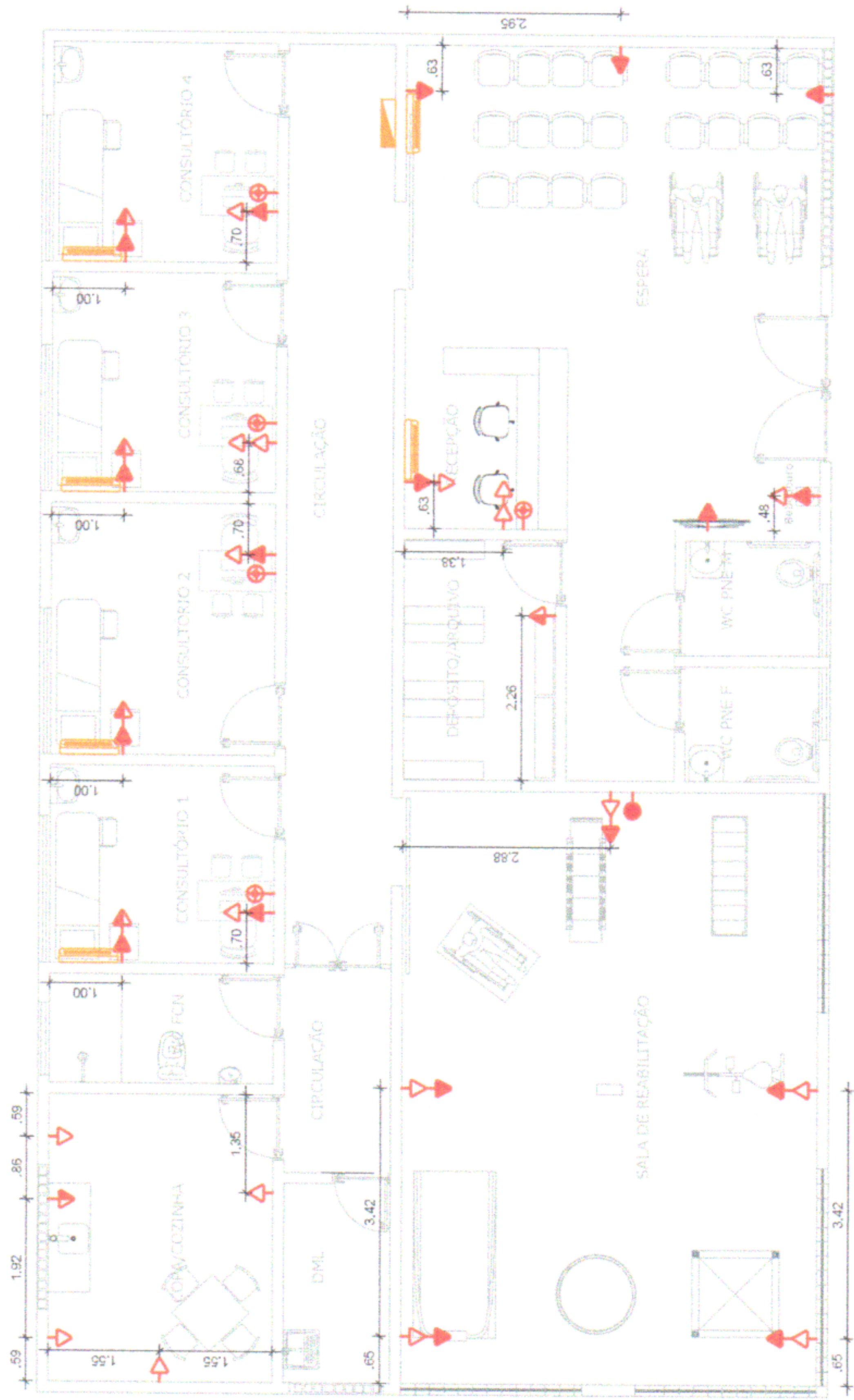
Planta baixa PONTOS DE ELÉTRICA
