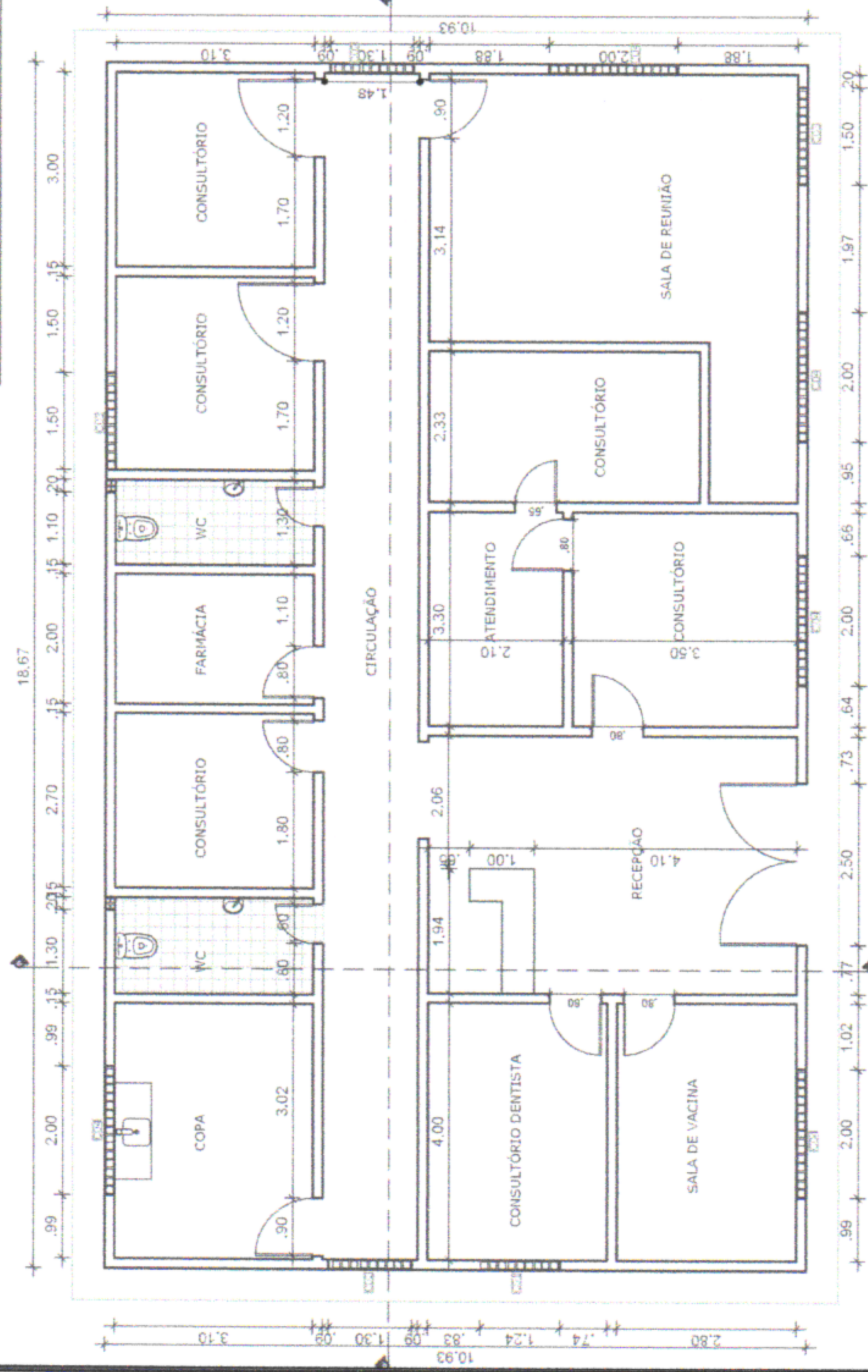
Planta baixa LEVANTAMENTO
