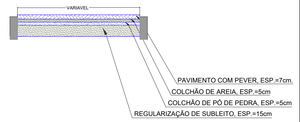
SEÇÃO TÍPICA DA 3ª TRAVESSA ALDERITA EVANGELISTA
