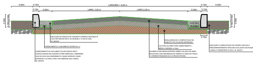
SEÇÃO TIPO DE PAVIMENTAÇÃO EM PARALELEPÍPEDOS DA 4ª TRAVESSA ADERITA EVANGELISTA
