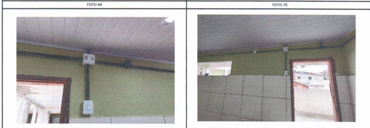
ESCOLA MUNICIPAL MARIA JOSÉ DE SOUZA - INSTALAÇÃO DE KIT ARSTOP COM DISJUNTOR 20A ESCOLA MUNICIPAL MARIA JOSÉ DE SOUZA - INSTALAÇÃO DE KIT ARSTOP COM DISJUNTOR 20A
