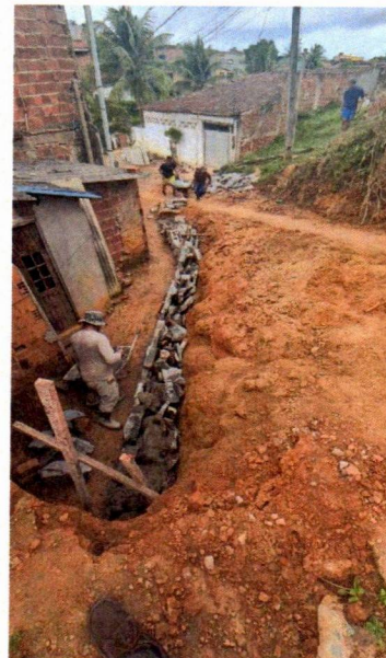
(08) Base do Muro
