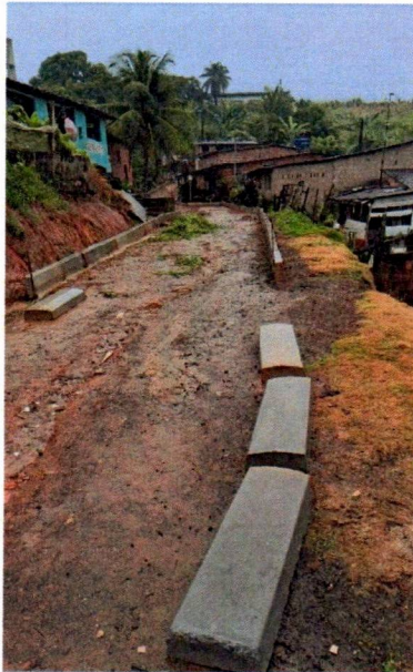
(05) Assentamento de meio-fio
