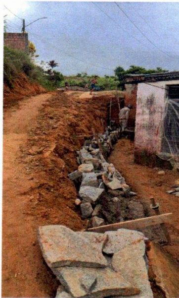
(07) Base do Muro
