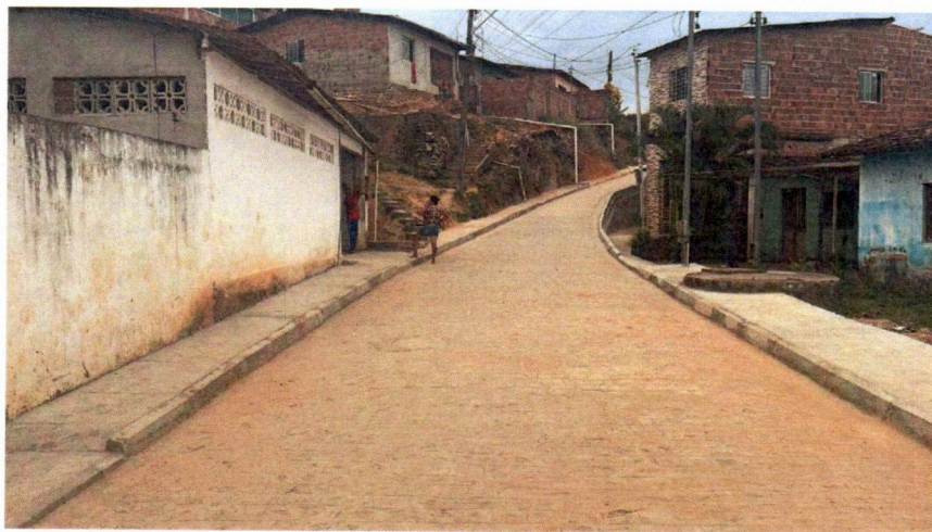
(16) Pavimentação em Paralelo
